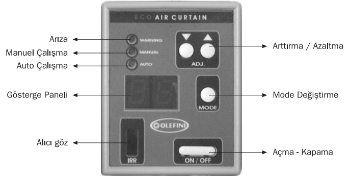
Şekil 1 Kontrol Paneli
