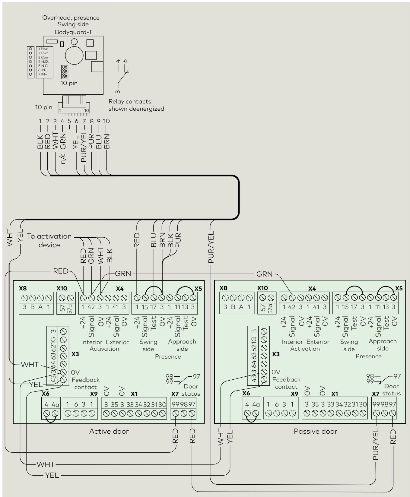
FIG. A3.2.1 BEA Bodyguard-T wiring, double door
