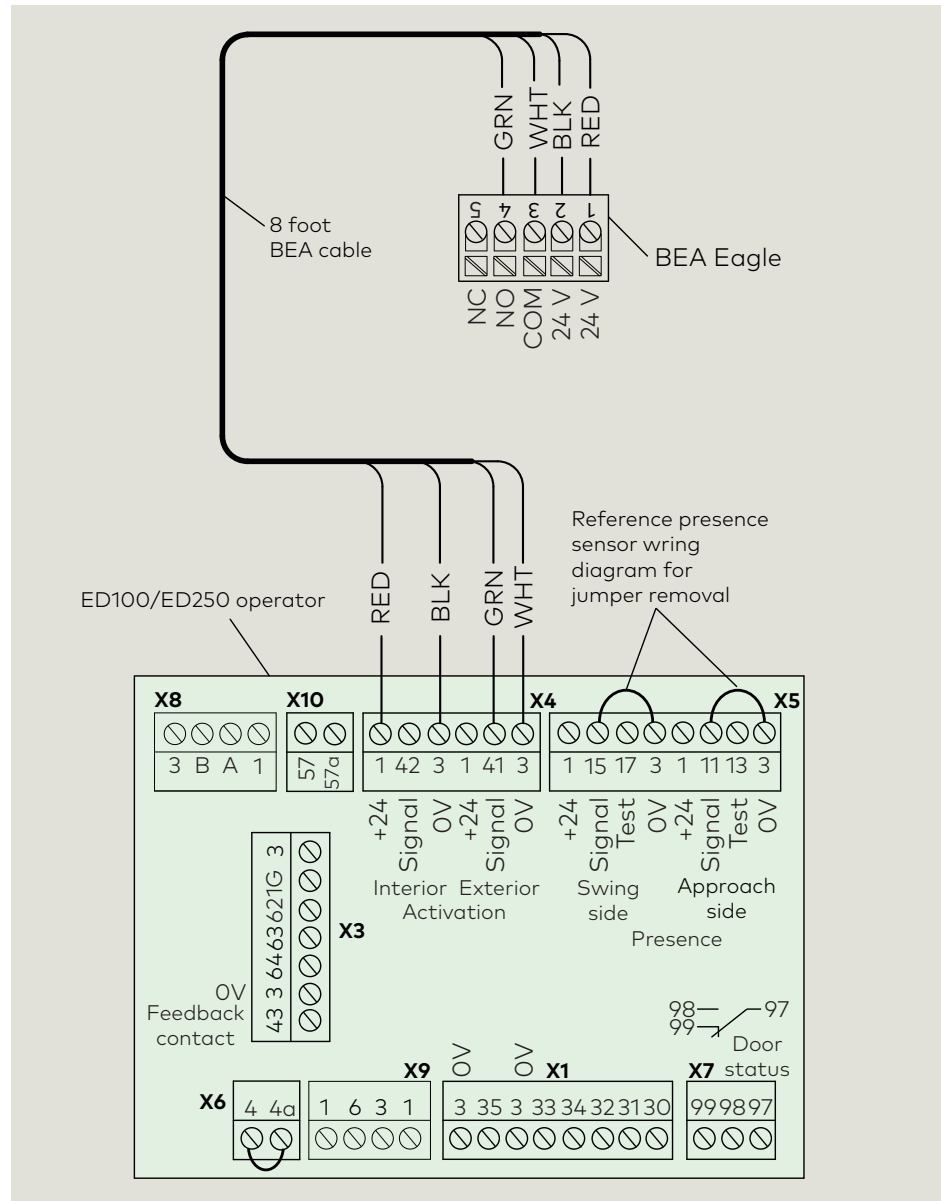
FIG. A4.1.1 BEA Eagle wiring
