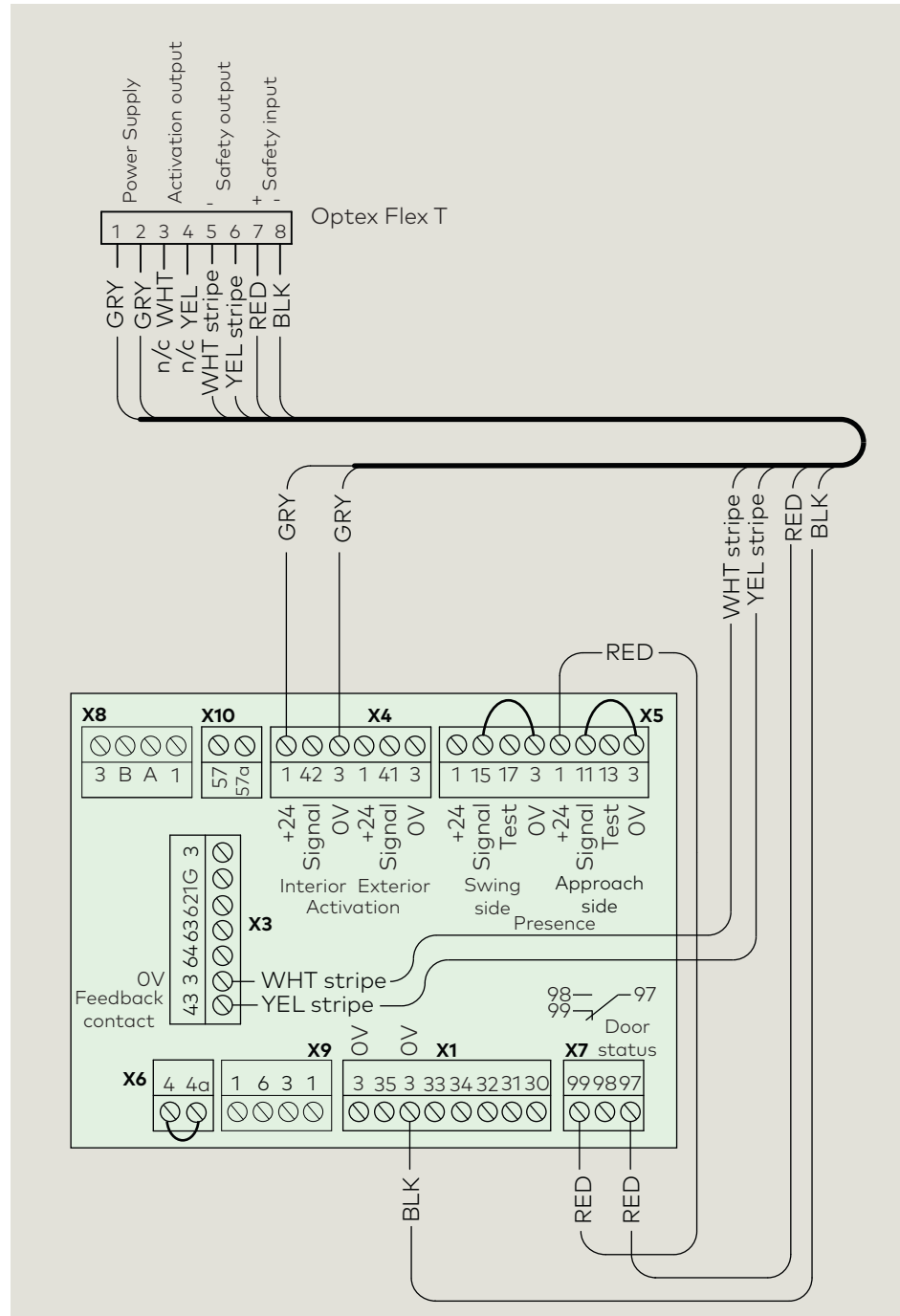
Fig. A8.1.1 Optex Flex T sensor wiring
